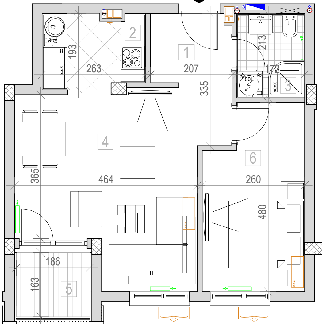
osnova stana br. 26 IV sprat
